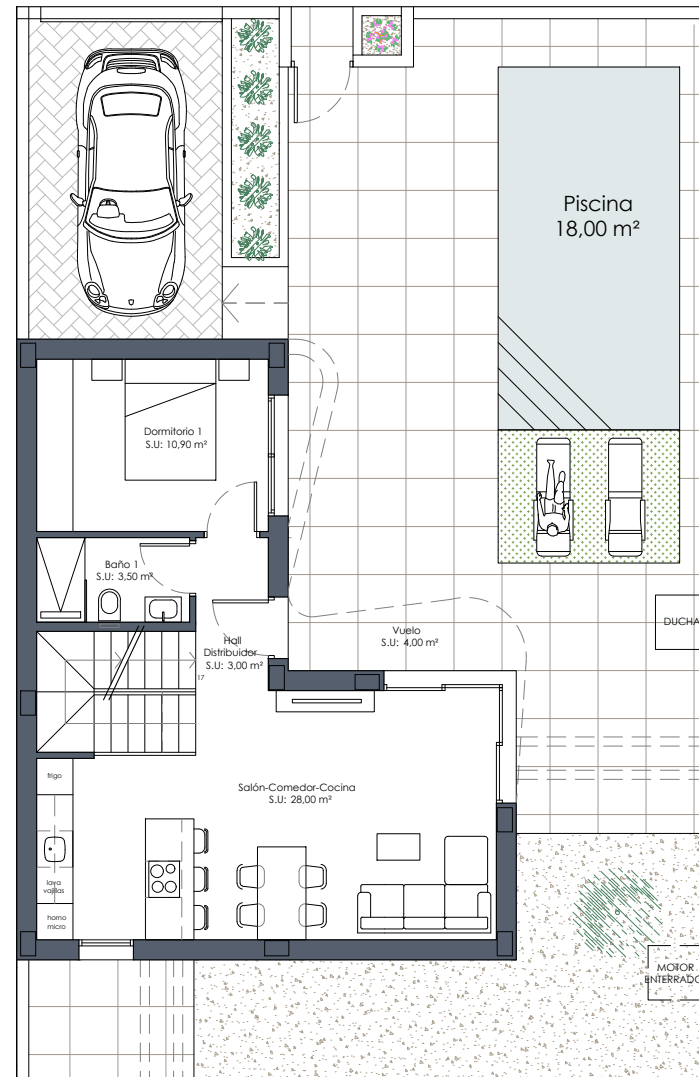
PLANTA BAJA
