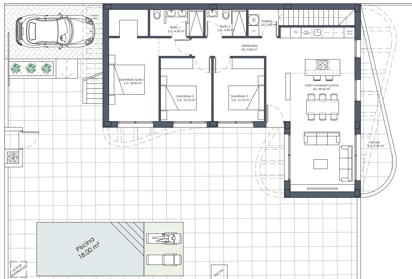
PLANTA BAJA
