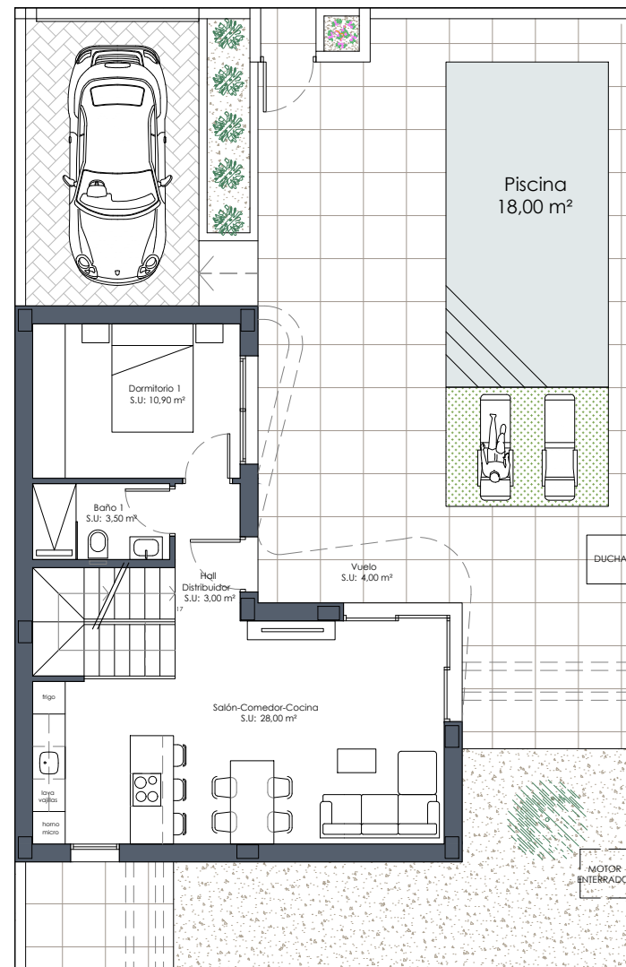
PLANTA BAJA
