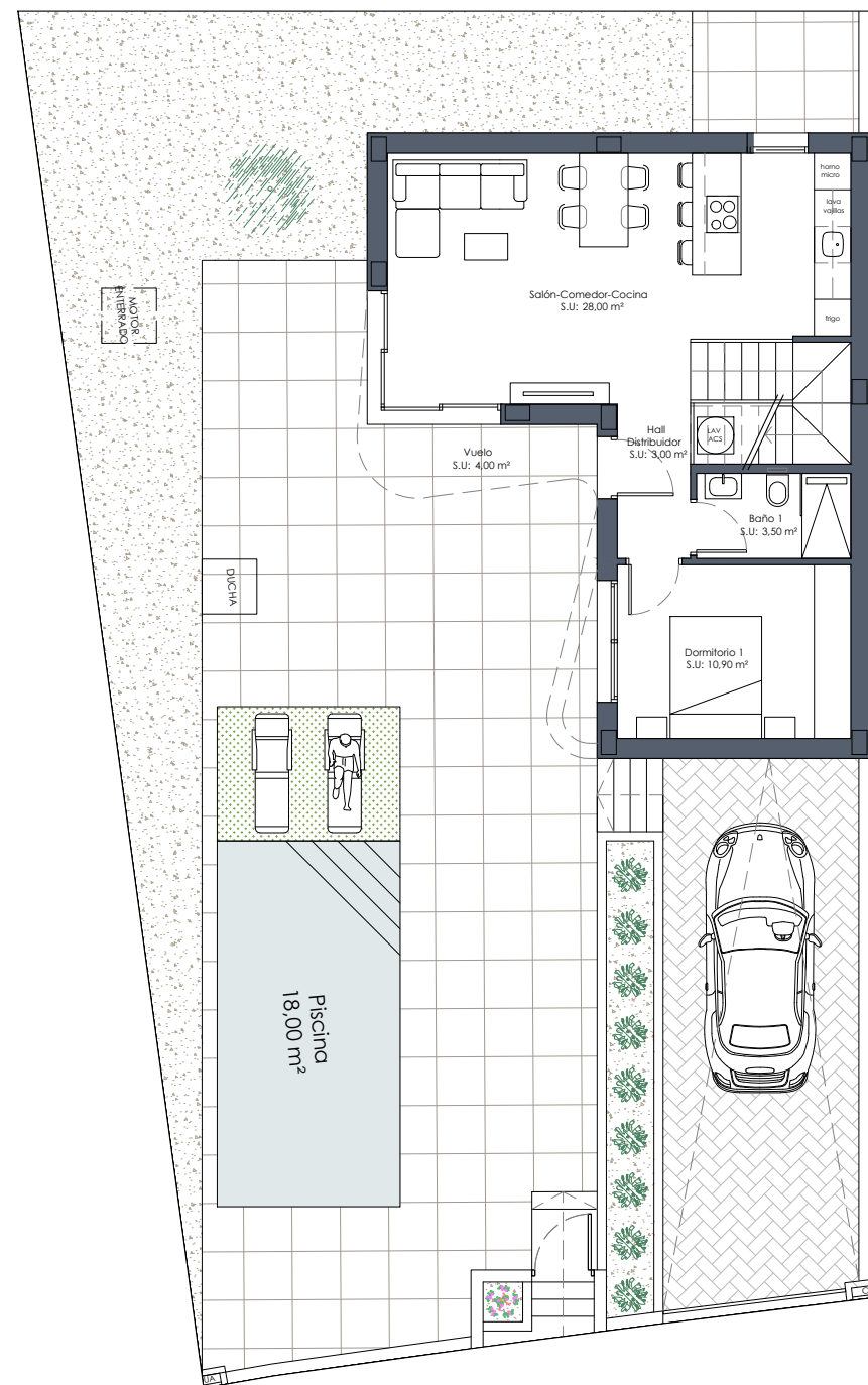
PLANTA BAJA
