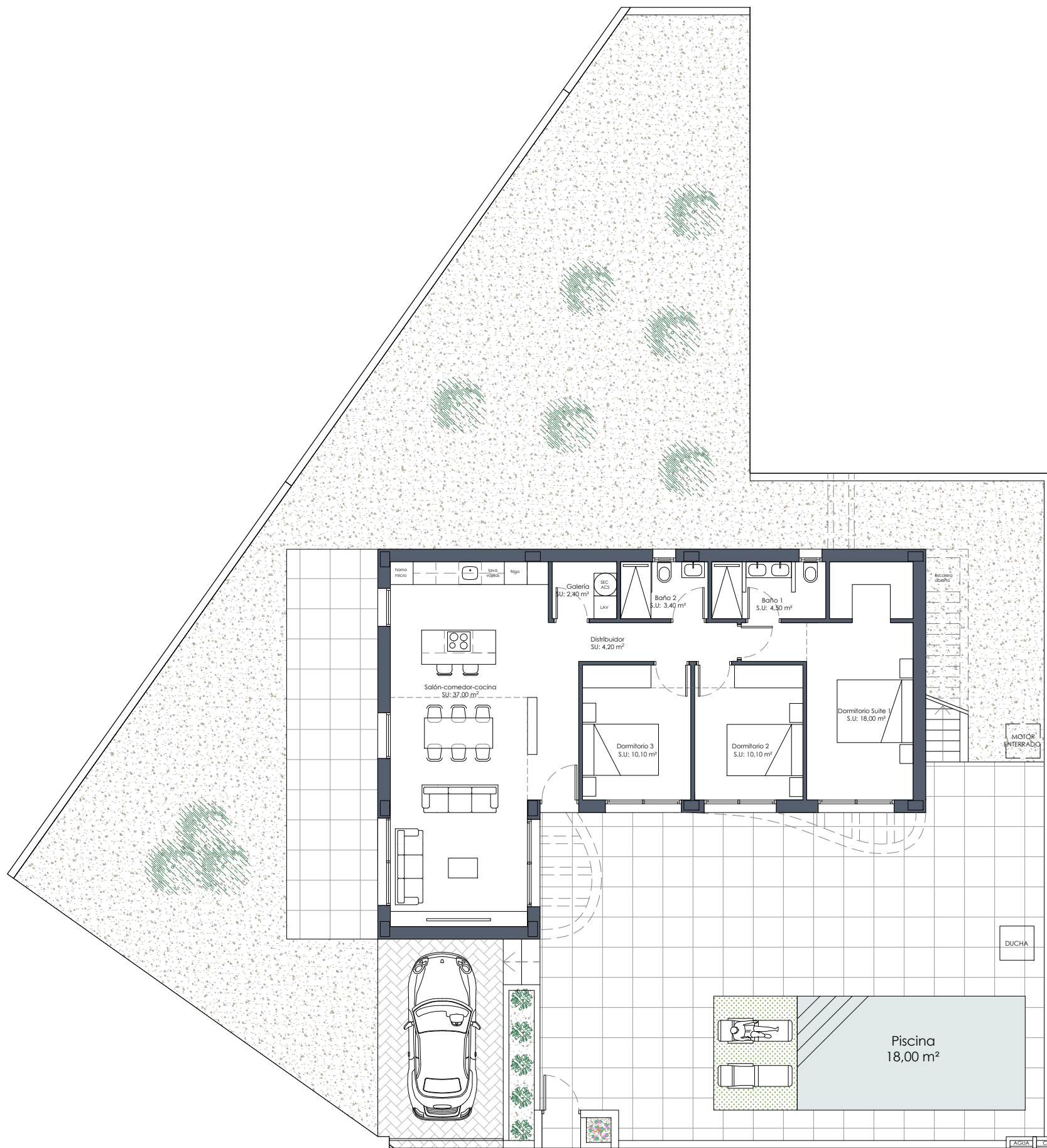
PLANTA BAJA
