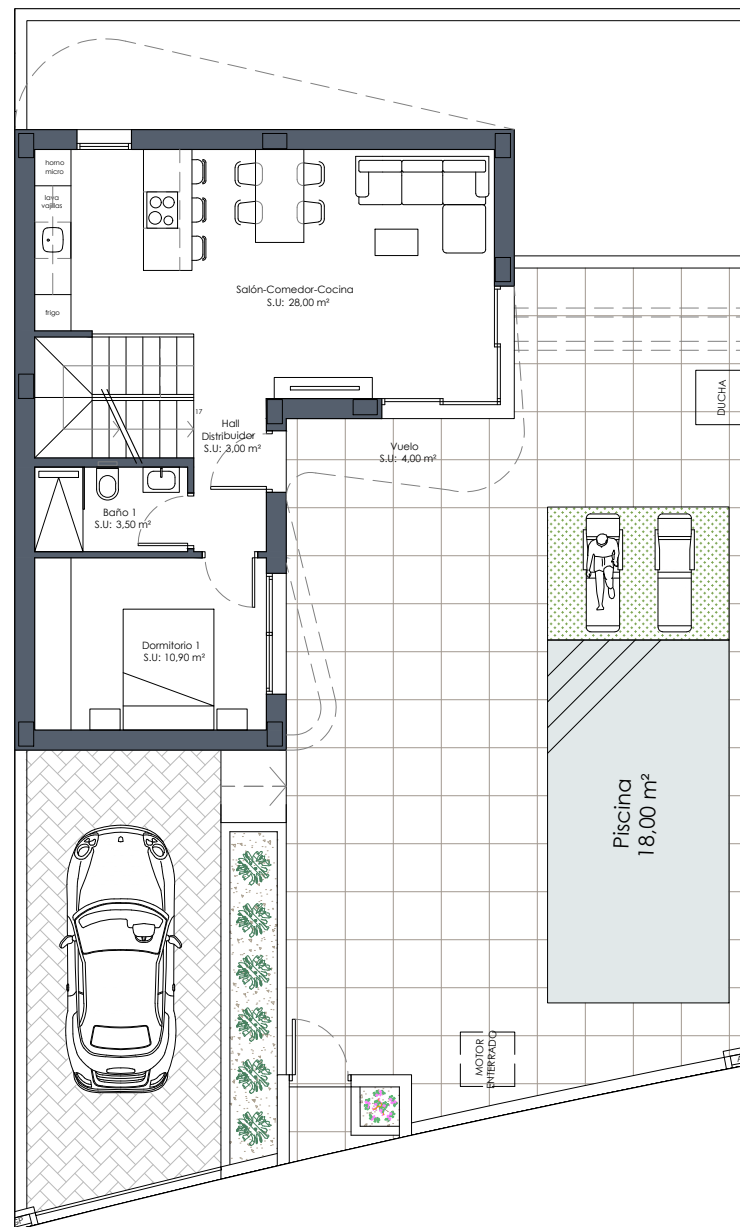
PLANTA BAJA
