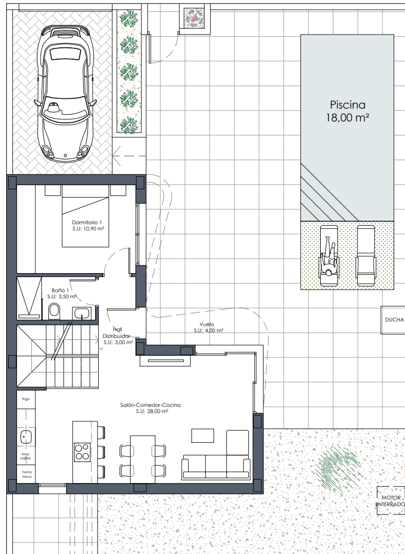
PLANTA BAJA
