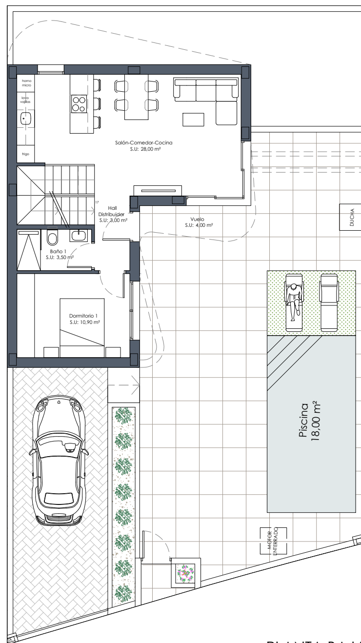
PLANTA BAJA
