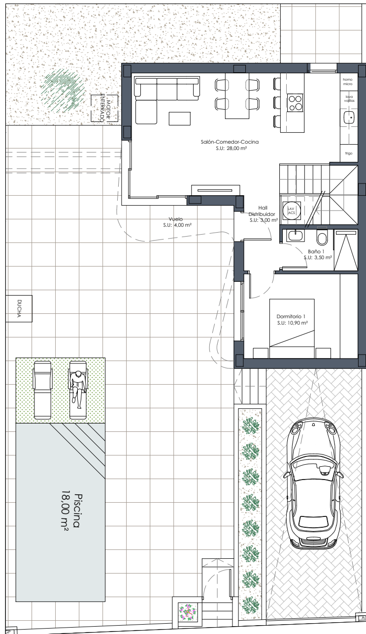
PLANTA BAJA
