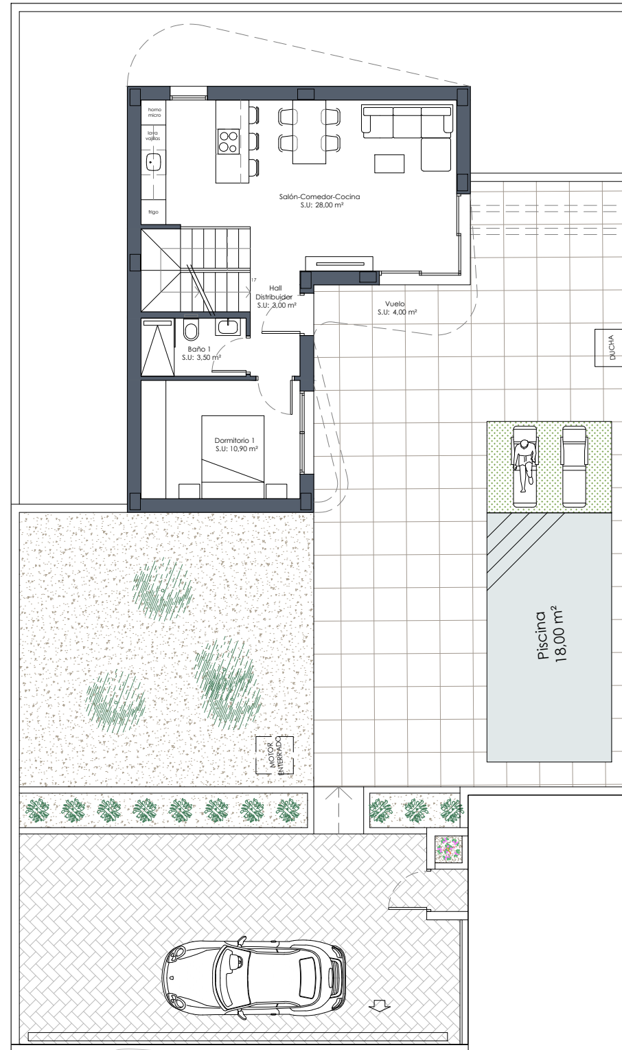
PLANTA BAJA
